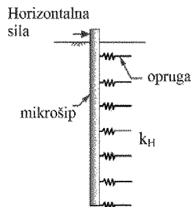
Slika 4. Mikrošip opterećen horizontalnom silom Figure 4. Micropil loaded with horizontal force
