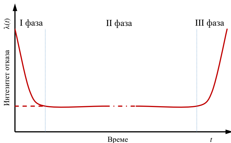
Слика 4.1.1. Упростијени приказ промене интензитета отказа у времену (bathtub curve)
