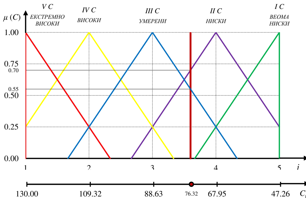
Слика 8.2.2.3.2. Процес фазификације трошкова – примена методе тежисита за оцену економских показатеља - дозер А3
