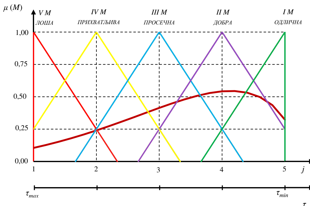
Слика 7.2.1.3. Процес мапирања функције густине времена одржавања на фази скупове погодности одржавања
