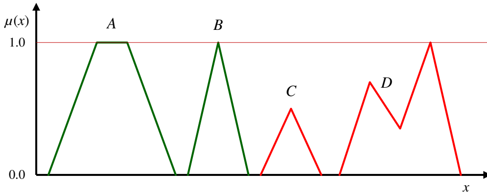
Слика 6.2.1.8. Фази скупови и испуњеност услова за фази број: A и B јесу фази бројеви; C не испуњава услов нормалности; D не испуњава услов конвексности, [115]
