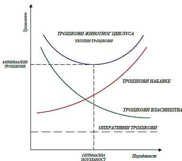
Слика 4.2.1. Однос трошкова животног циклуса и поузданости, оптимално време за замену техничког система, према IEC 300-3-3, [66]
