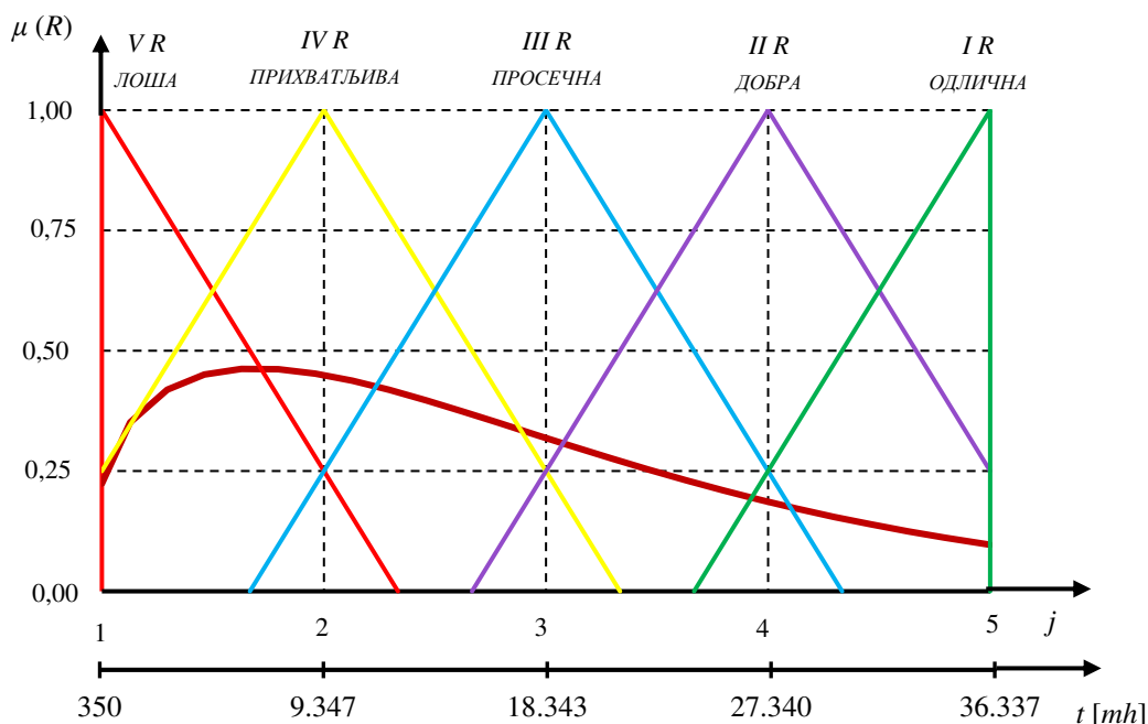
Слика 8.1.2.1. Процес мапирања функције густине отказа на фази скупове поузданости – дозера A1
