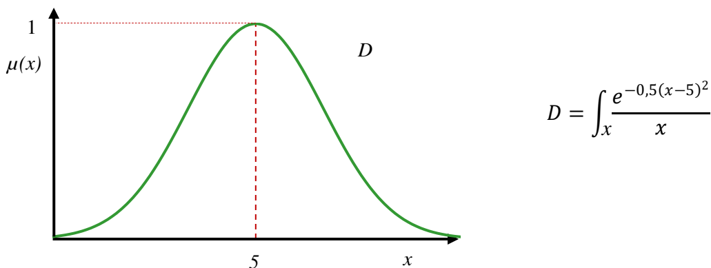
Слика 6.2.1.1. Облици фази функција припадности према [112]:
