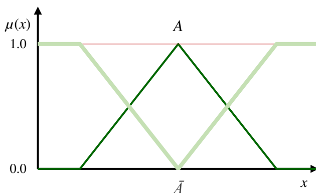
Слика 6.2.1.6. Комплемент фази скупа A , [113] и др.
