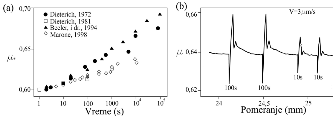
Slika 4-9. a) Promene vrednosti statičkog trenja u funkciji vremena kontakta dva bloka za inicijalno uglaçane površine stenske mase (tamni simboli) i zdrobljeni kataklastični materijal (svetli simboli); b) Dijagram trenje-pomeranje koji ilustruje promenu koeficijenta statičkog trenja pri trzanju. Vreme statičkog kontakta (u stanju mirovanja blokova) izraženo je u sekundama, a brzina smicanja je 3\mu\text{m/s} [Marone, 1998]
