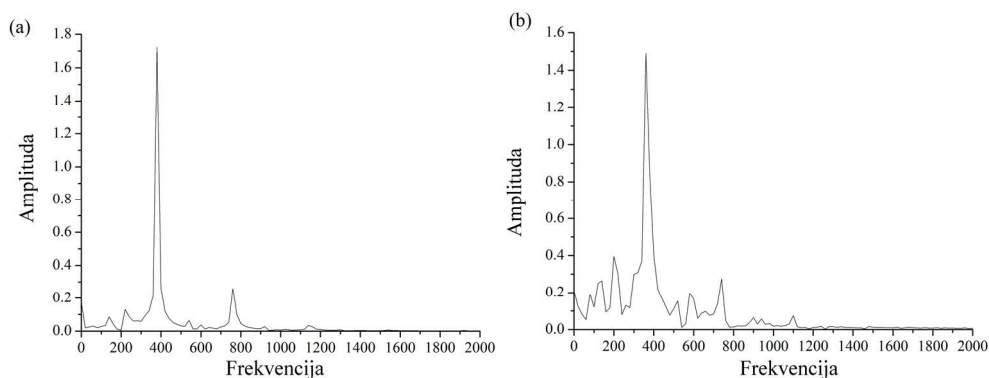
Slika 7-60. Furijeov spektrar snage za vremenske serije prikazane na slici 7-59: (a) dva izražena pika u spektru snage za vremensku seriju na slici 7-59(1) ukazuju na pojavu kvaziperiodičnog ponašanja u modelu; (b) širokopojasni kontinualni šum u Furijeovom spektru snage za vremensku seriju sa slike 7-59(2) ukazuje na determinističko haotično ponašanje u modelu.
