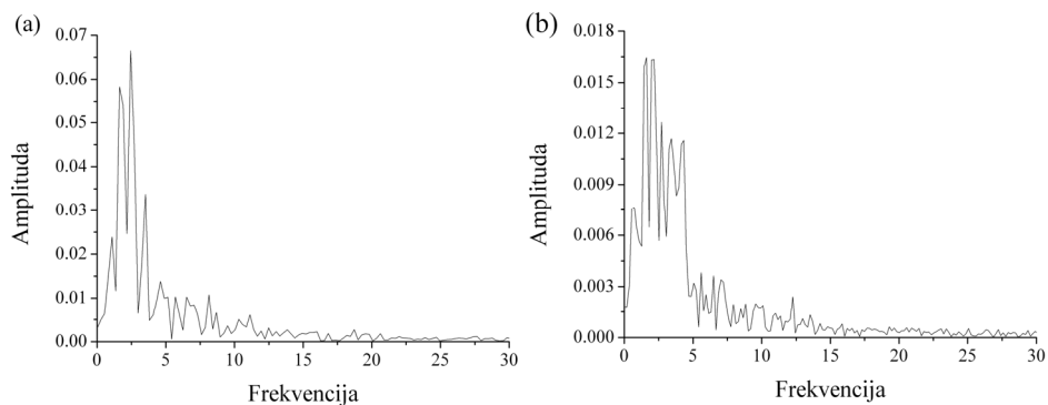
Slika 2. Furijeov spektar snage za ubrzanje tla za vreme potresa magnitude M \approx 1,5 ( E=1 \times 10^7 \text{J} ) izazvanog rudarskim aktivnostima u basenu uglja u Gornjoj Sileziji u (a) horizontalnom (sever-jug) i (b) vertikalnom pravcu. Kvalitativno sličan spektar snage se dobija i za ubrzanje tla u horizontalnom pravcu istok-zapad. Kontinualni spektar snage u oba slučaja ukazuje ili na moguće deterministički haotično ili na nasumično ponašanje posmatranog sistema.
