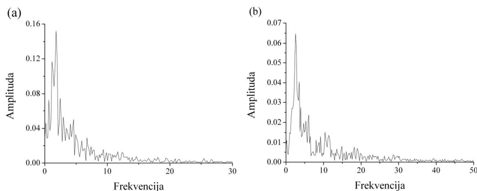
Slika 2. Furijeov spektar snage za ubrzanje tla registrovano za vreme potresa M \approx 2 ( E=5 \times 10^7 \text{J} ) izazvanog rudarskim aktivnostima u basenu bakra Legnica-Glogov u (a) horizontalnom (sever-jug) i (b) vertikalnom pravcu. Kvalitativno sličan spektar snage se dobija i za ubrzanje tla u horizontalnom pravcu (istok-zapad). Kontinualni spektar snage u oba slučaja ukazuje ili na moguće deterministički haotično ili na nasumično ponašanje posmatranog sistema.
