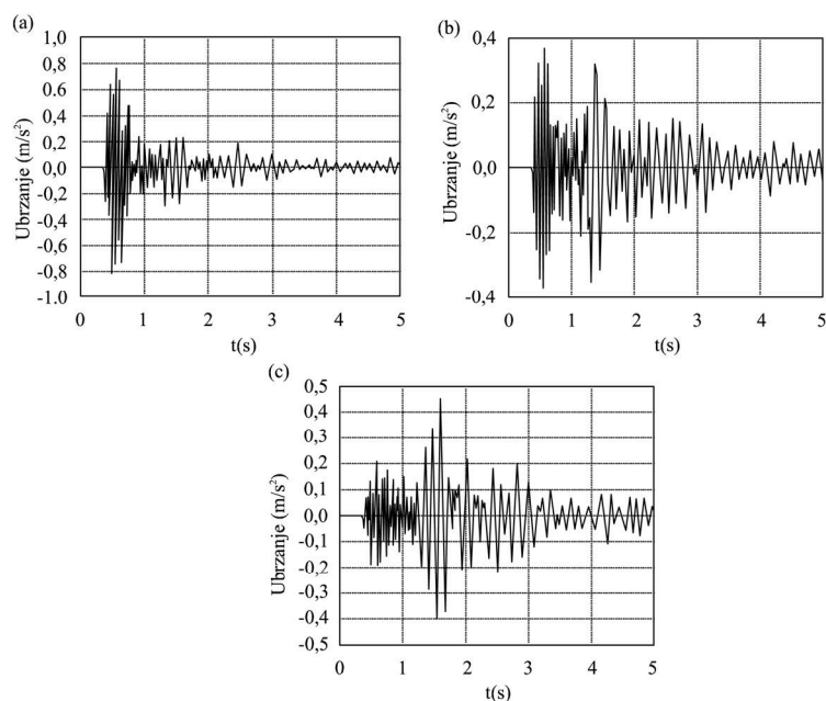
Slika 1. Vremenske serije tipičnog ubrzanja oscilovanja tla za vreme potresa M \approx 2 ( E=5 \times 10^7 \text{J} ) izazvanog rudarskim aktivnostima u basenu bakra Legnica-Glogov, u tri pravca: (a) – sever-jug (1236); (b) – istok zapad (1386) i (c) – vertikalno (1037) [Dulinska, Fabijanska, 2011].
