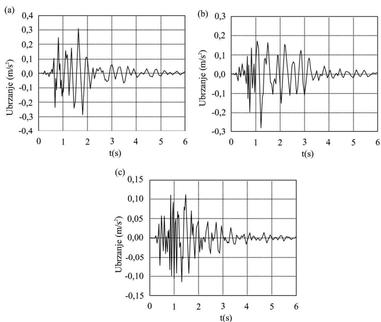
Slika 1. Vremenske serije tipičnog ubrzanja oscilovanja tla za vreme potresa magnitude M \approx 1,5 ( E=1 \times 10^7 \text{J} ) izazvanog rudarskim aktivnostima u basenu uglja u Gornjoj Sileziji, u tri pravca: (a) – sever-jug (748); (b) – istok zapad (865) i (c) – vertikalno (1126) [Dulinska, Fabijanska, 2011]
