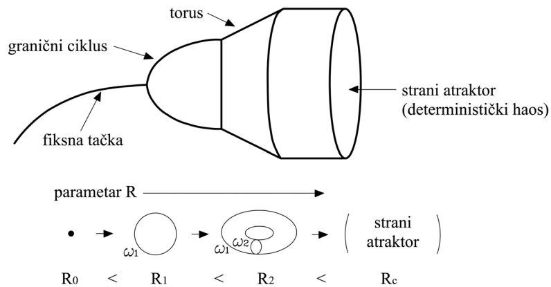
Slika 5-12. Ruel-Takens-Njuhaus put u kaos.
