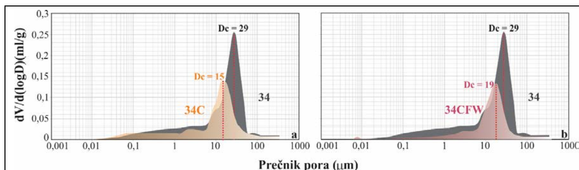
Sl. 77. Kriva distribucije veličine pora izražena logdiferencijalnom zapreminom u netretiranom i tretiranom uzorku grainstone ; a) uzorak 34 konsolidovan sa C ; b) uzorak 34 konsolidovan sa CFW
