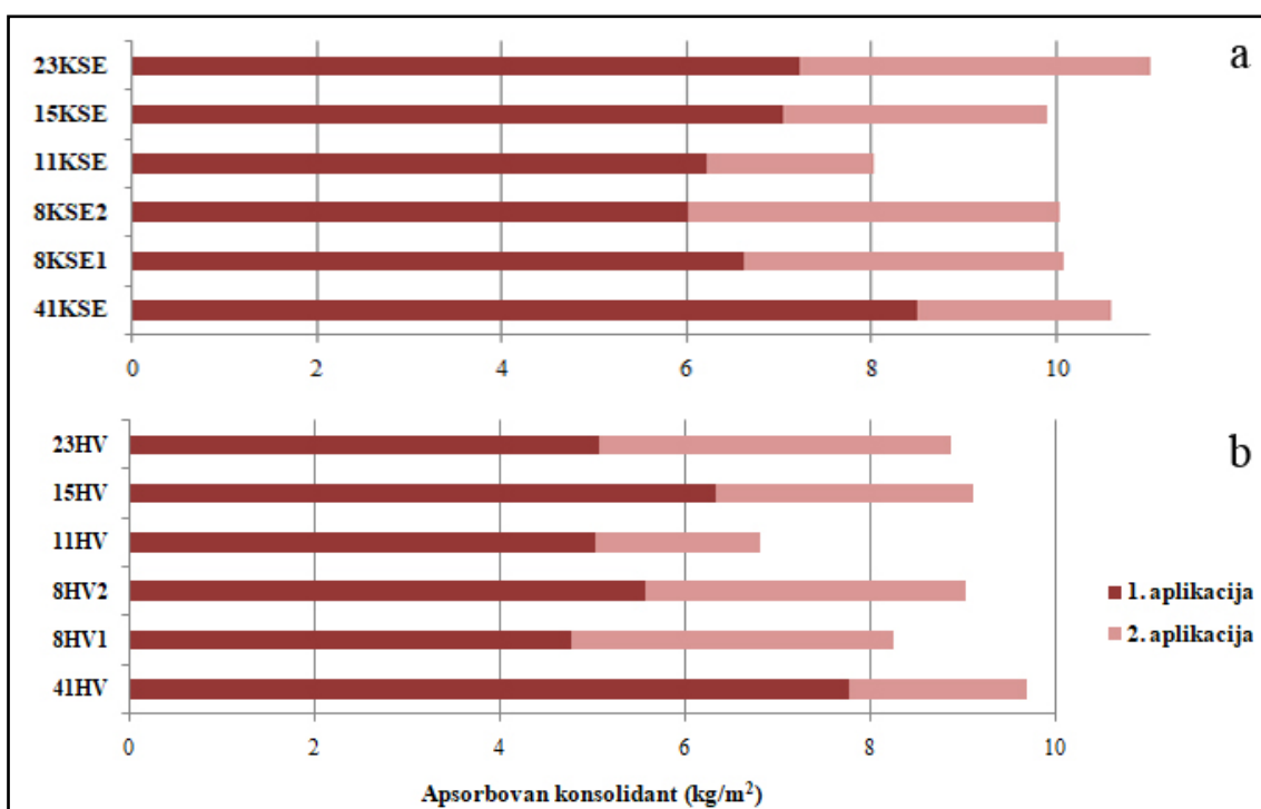
Sl. 97. Količine apsorbovanog konsolidanta KSE i HV pri aplikacijama u jednom ciklusu uzoraka algalnog rudstone
