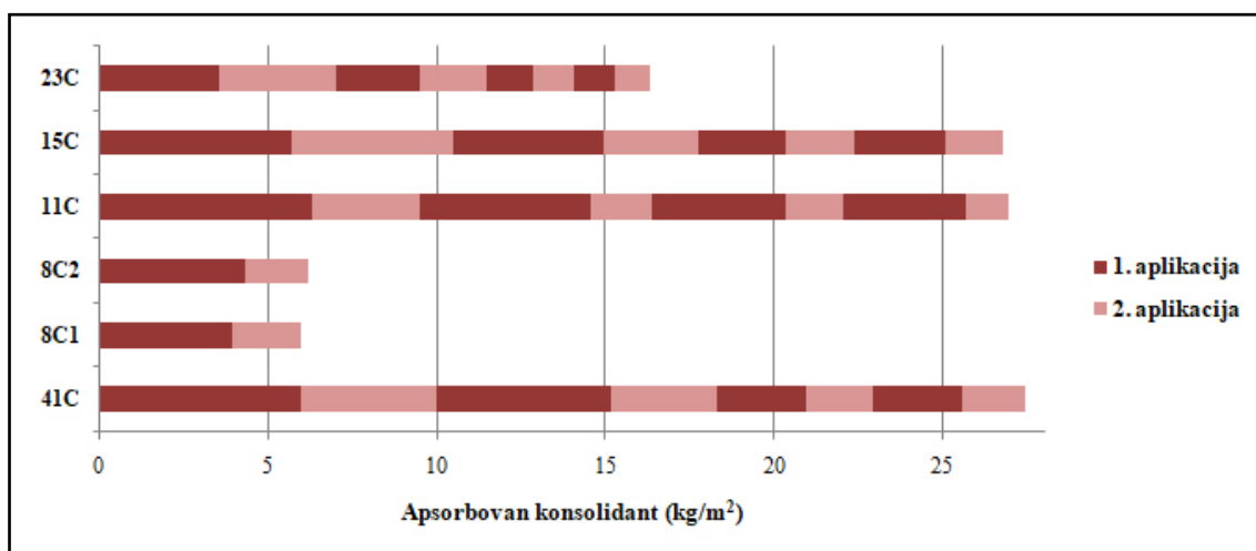
Sl. 95. Količine apsorbovanog konsolidanta C pri aplikacijama u četiri ciklusa uzoraka algalnog rudstone
