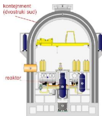
Slika 2 – Nuklearni reaktor tipa VVER-1200 [1]
