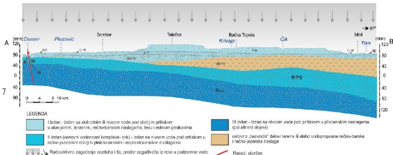
Slika 3 – Hidrogeološki profil (zapad-istok), od Dunava do Tise [2]
