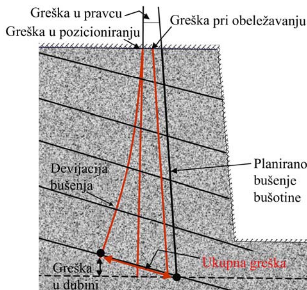
Slika 2-11. Različiti uzroci devijacije bušenja [53]
