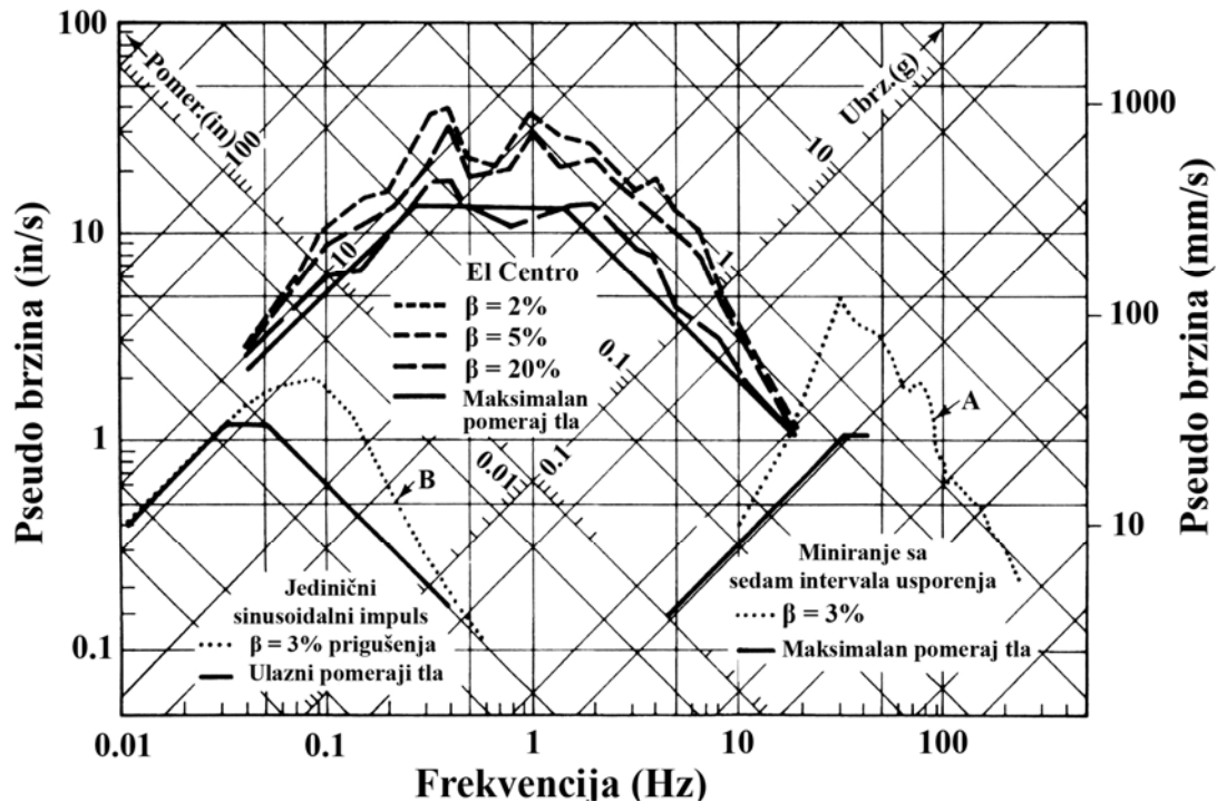
Slika 2-29. Spektri odziva pri zemljotresu, jednom sinusoidalnom impulsu i miniranjuna površinskom kopu sa sedam intervala usporenja ( \beta = 3\% ) [48]
