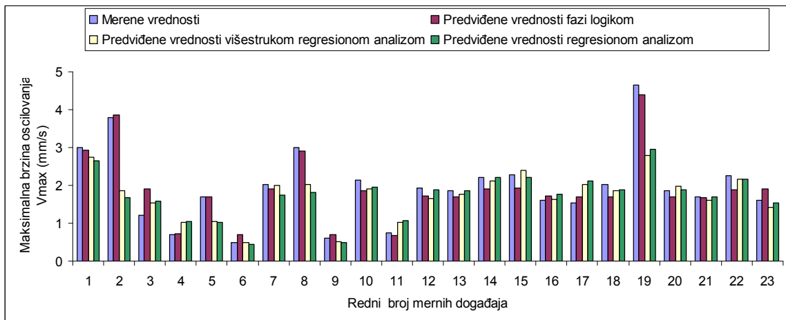
Slika 5-61. Razlika vrednosti maksimalne brzine oscilovanja tla dobijene analizoum podataka sa terena i predviđenih dobijenih višestrukoum regresionoum analizoum, prostoum regresionoum analizoum i fazi modeloum
