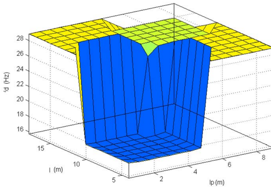
Slika 5-36. 3D prikaz dominantne frekvencije f_d u odnosu na dužinu minske bušotine l i dužinu minskog punjenja l_p
