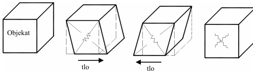
Slika 2-37. Vibraciona ili „X“ pukotina [42]
