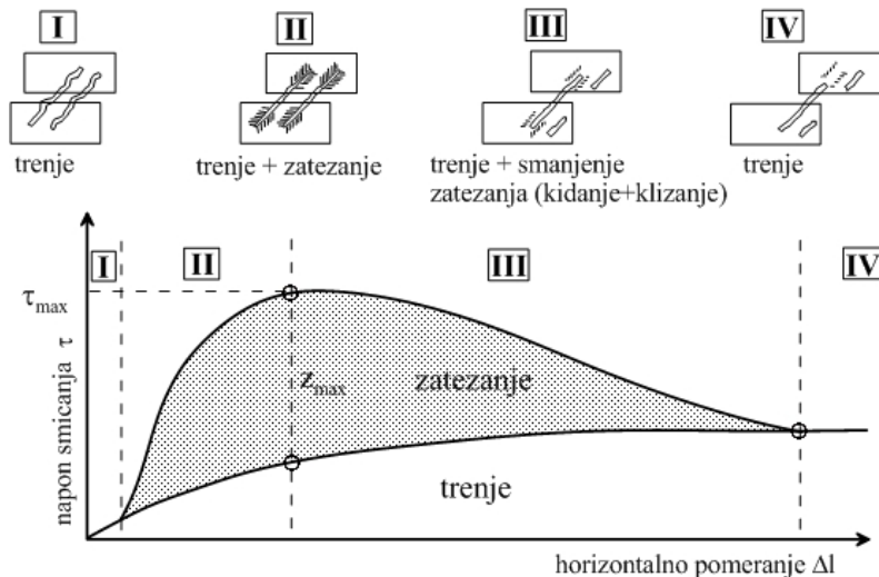
Slika 6.14. Ponašanje komunalnog otpada pri opitu smicanja (Kölsch, 1996)
