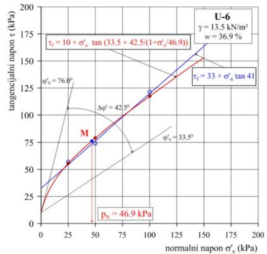
Slika 6.130 Čvrstoća smicanja za krivolinijsku jednačinu loma hiperboličkog oblika (uzorci iz serije B, c' = 10 kPa)
