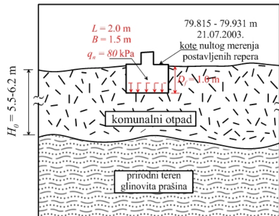
Slika 9.16. Opšti geotehnički model terena u zoni objekta
