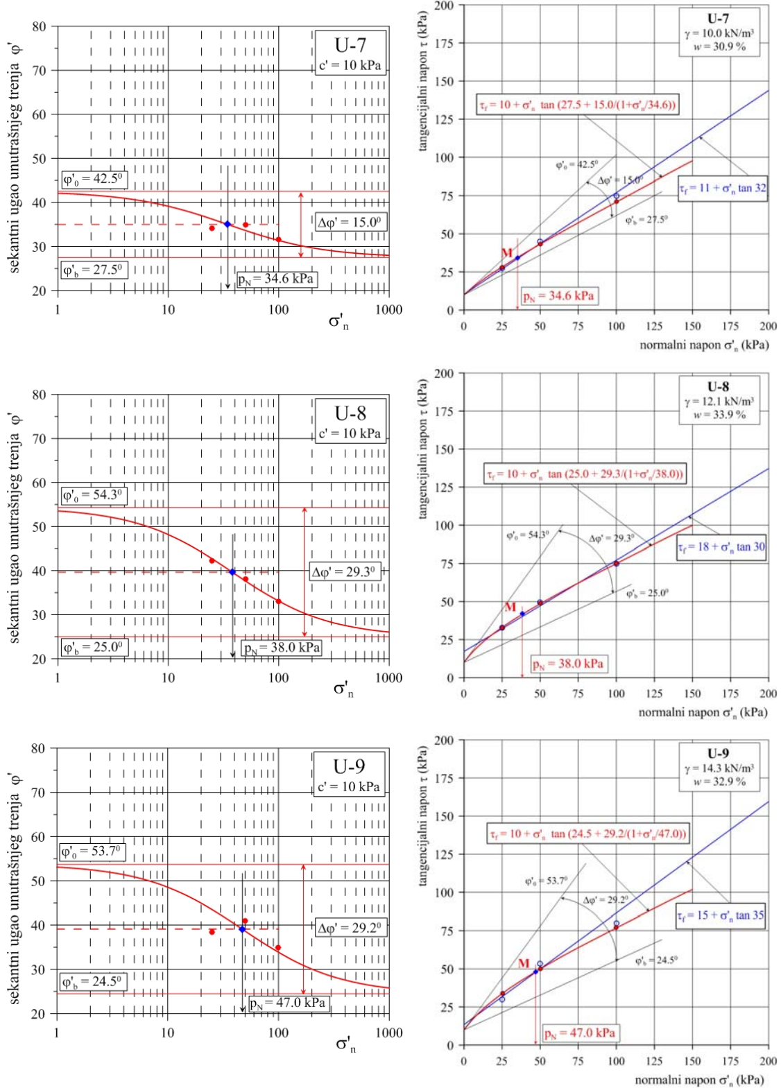
Slika 6.133 Čvrstoća smicanja za krivolinijsku jednačinu loma hiperboličkog oblika (uzorci iz serije C, c' = 10 kPa)
