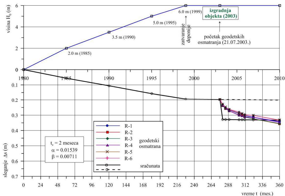
Slika 9.22. Poređenje sračunatih i izmerenih vrednosti sleganja – logaritamska funkcija
