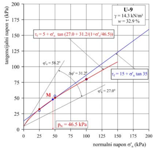
Slika 6.132 Čvrstoća smicanja za krivolinijsku jednačinu loma hiperboličkog oblika (uzorci iz serije C, c' = 5 \text{ kPa} )
