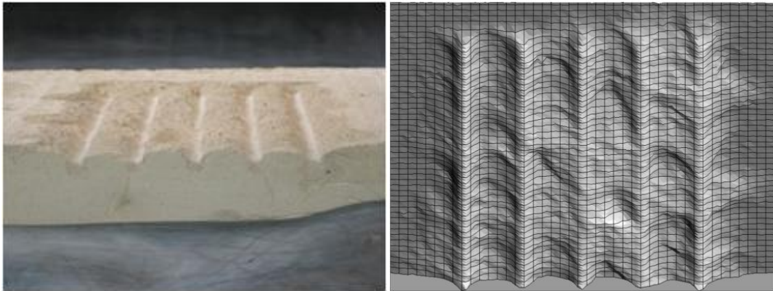
Slika 2.8. Izgled površine i model površine testiranog uzorka
