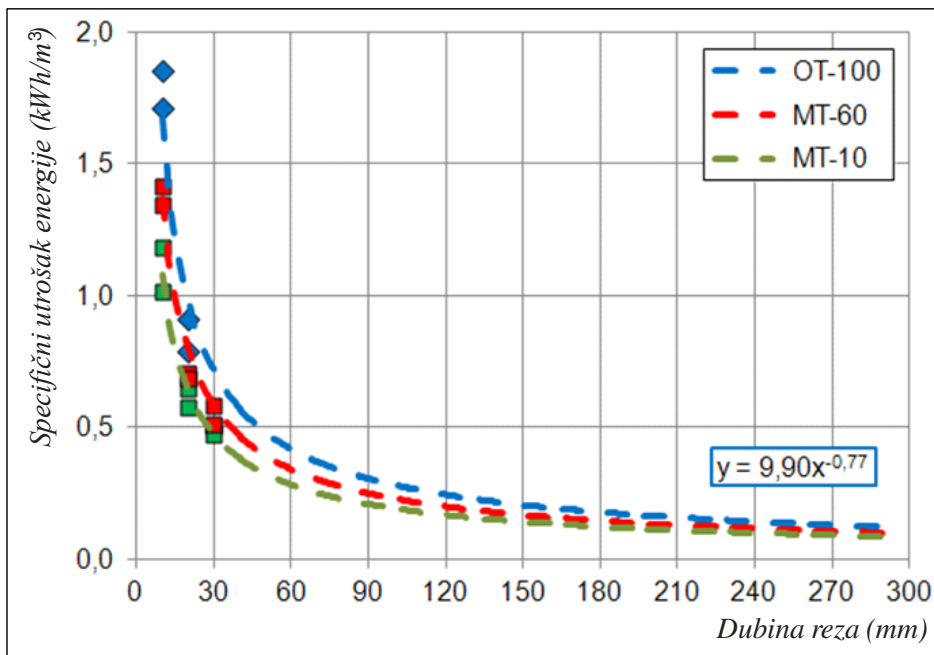
Slika 2.16. Uticaj debljine reza na specifičnu potrošnju energije
