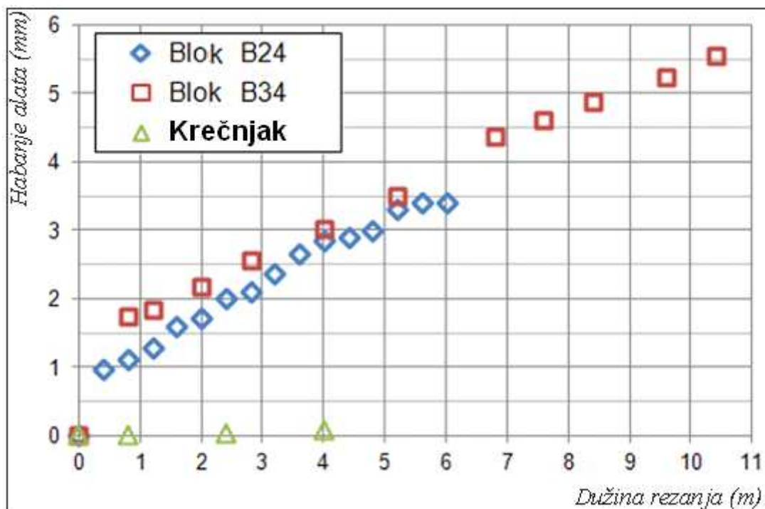
Slika 2.6. Habanje alata (zuba) u zavisnosti od debljine reza i vrste stenskog materijala
