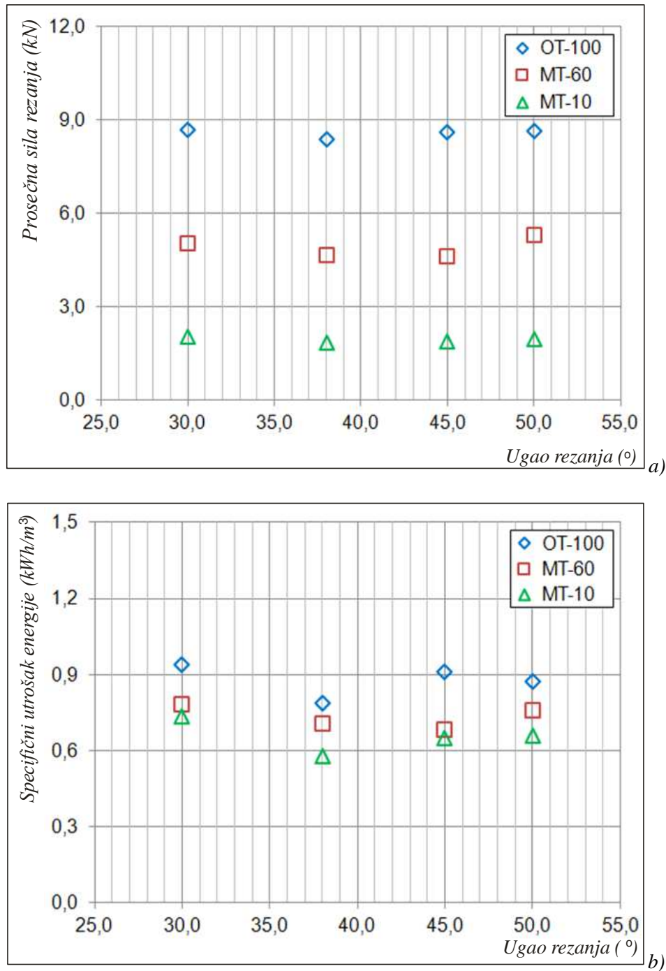
Slika 2.12. Uticaj ugla rezanja na: a) reznu silu i b) specifičnu potrošnju energije
