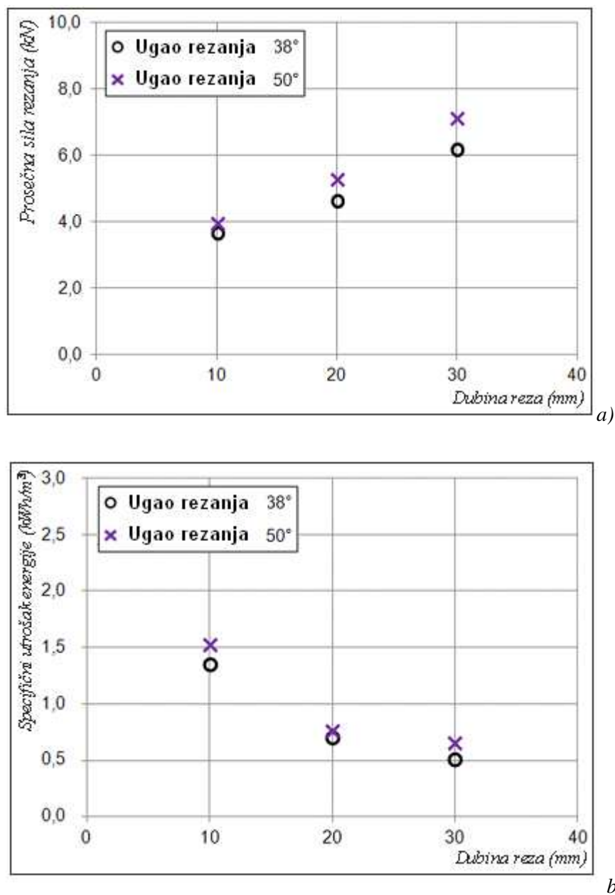
Slika 2.13. Uticaj debljine reza na: a) reznu silu i b) specifičnu potrošnju energije
