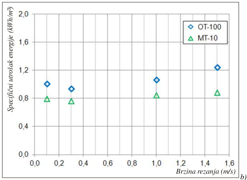
Slika 2.11. Uticaj brzine rezanja na: a) reznu silu i b) specifičnu potrošnju energije
