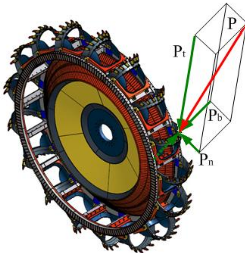
Slika 3.24. Sile koje deluju na vedricu pri otkopavanju materijala ( P – rezultanta sile kopanja, P_t – tangentsna sila kopanja, P_b – bočna sila kopanja, P_n – normalna sila kopanja)
