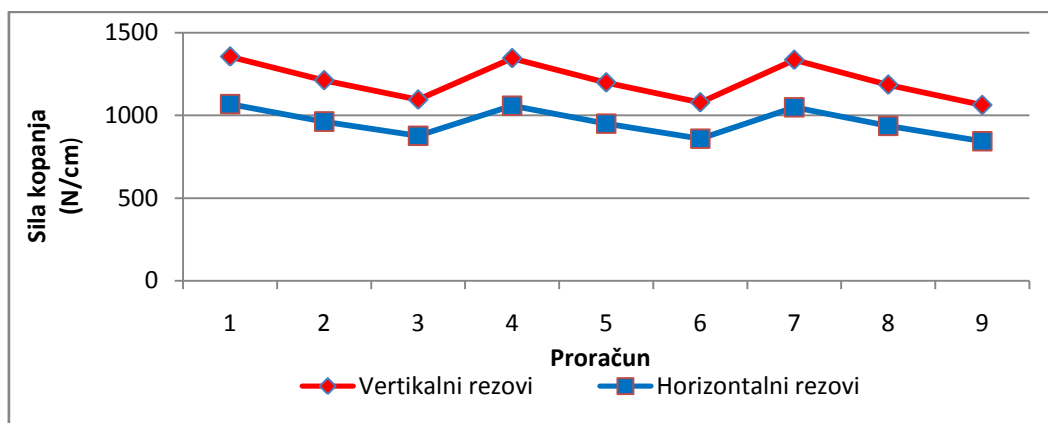
Slika 4.6. Uporedni dijagram raspoložive sile kopanja pri radu sa horizontalnim i vertikalnim rezovima
