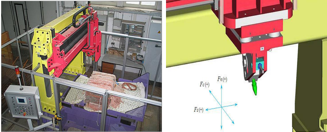
Slika 2.7. Aparatura HXS 1000-50 za merenje rezne sile
