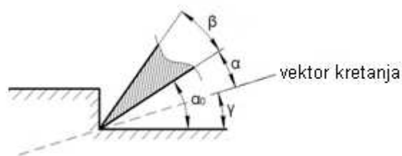
Slika 2.18. Šema za kinamtski proračun: a) prikaz preseka rotora; b) prikaz odozgo;
