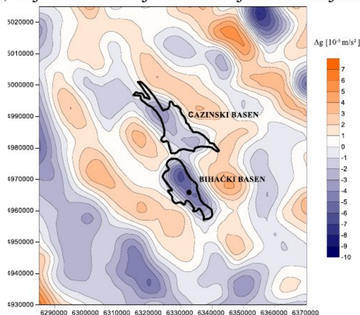
Slika 3 – Karta filtriranih lokalnih gravimetrijskih anomalija sa prikazanim položajem Bihaćkog i Cazinskog bazena
